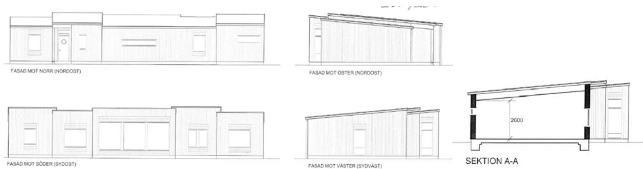
Fasad och sektionsritningar för nytt fritidshus
